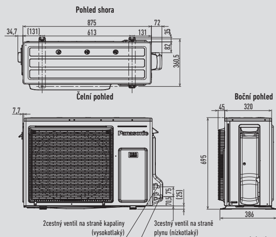
CU-Z50TKEA // CU-Z71TKEA
