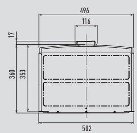
Pohled shora
