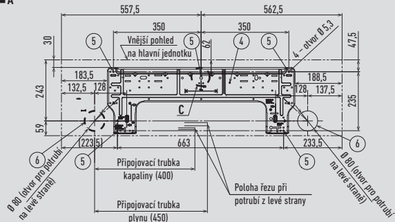
Pohled A
