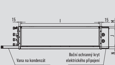
Zadní pohled
