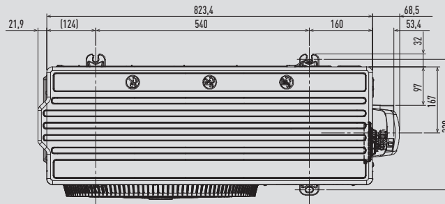
Pohled shora
