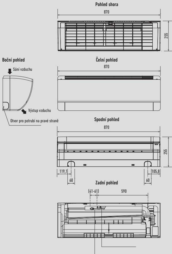
CS-E9PKEA // CS-E12PKEA
