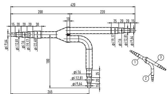
Kapalinové potrubí
