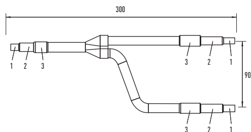
Kapalinové potrubí
