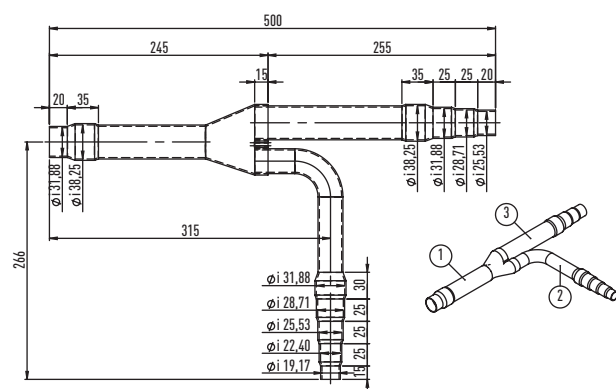
Plynové potrubí
